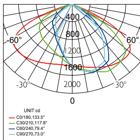
Curva fotométrica 400W
