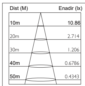
Curva luxométrica 100W
